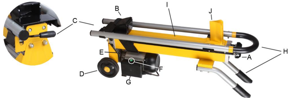
Fig. 1 Vue d'ensemble des composants principaux. Vérifier tous les composants selon la liste suivante, en se référant à l'illustration ci-dessus.
