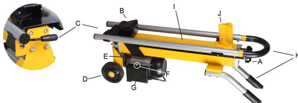
Fig. 1 Oversigt over de væsentlige komponenter
