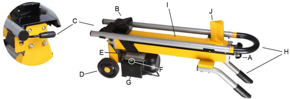
Abb. 1 Übersicht der wesentlichen Komponenten. Überprüfen Sie alle Komponenten entsprechend folgender Übersicht (Abb. 1).
