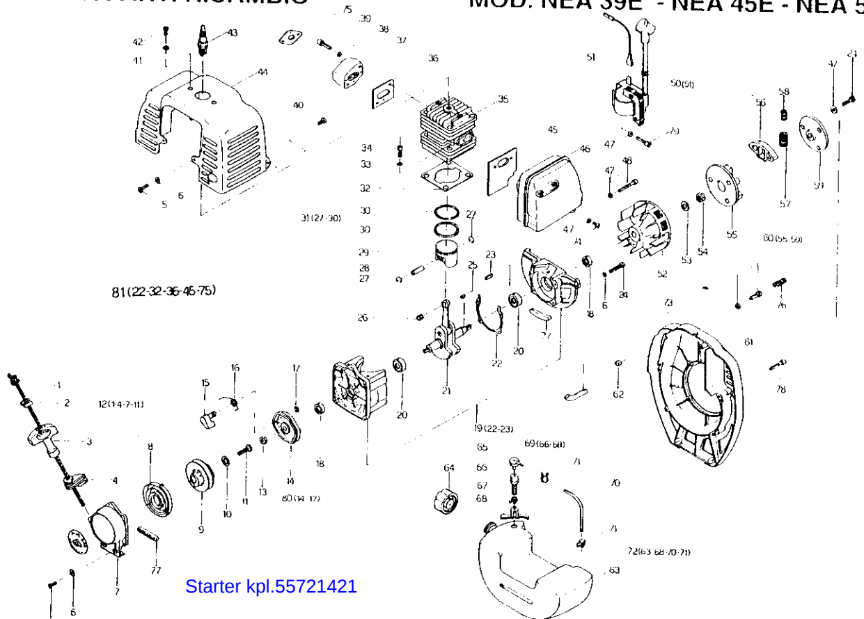
Fig 8 - Engine - moteur - Motore
